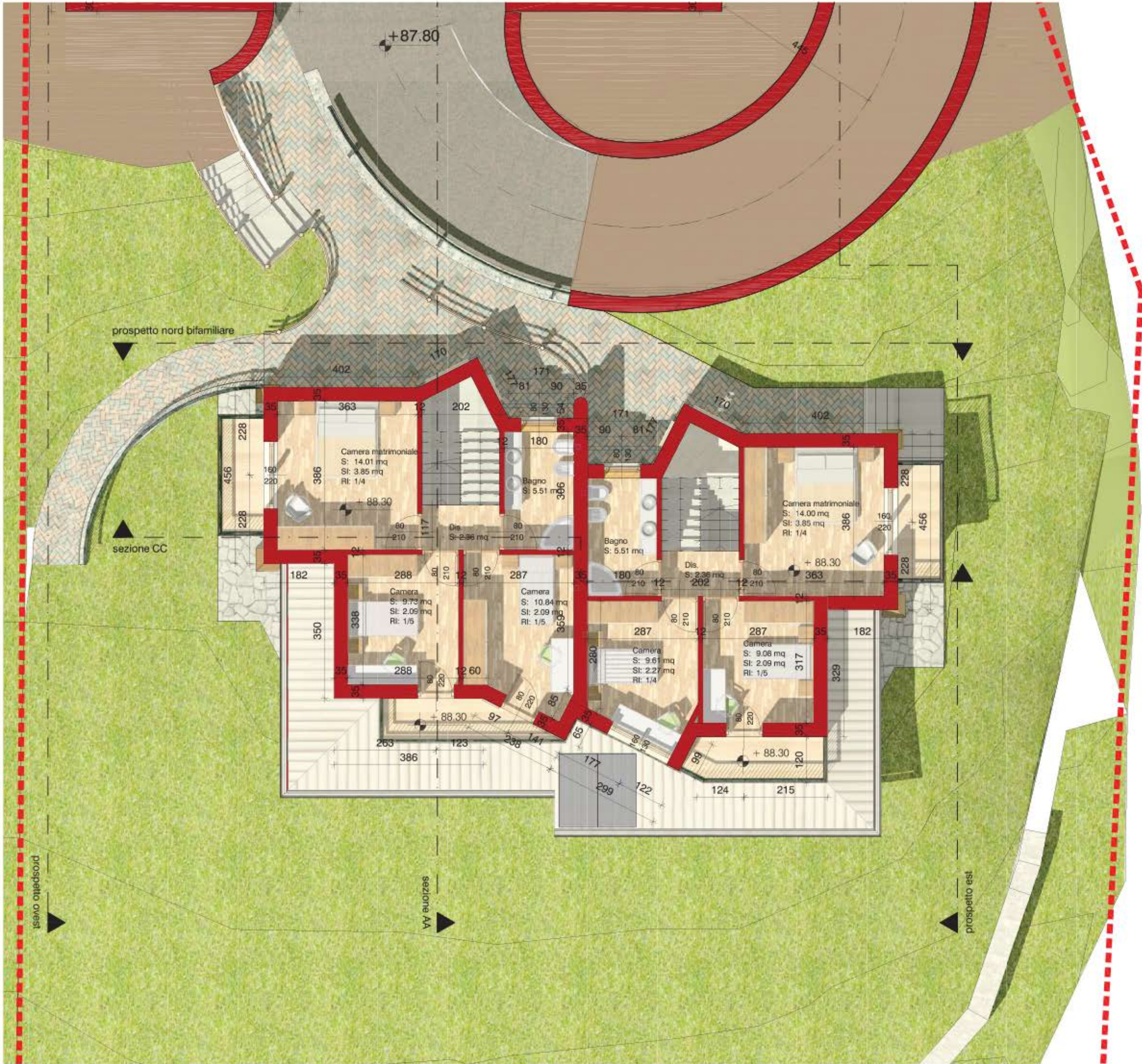
Pianta Piano Primo villa bifamiliare unità 2/3
